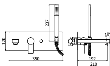
TA 001CR Miscelatore incasso vasca/doccia completo di deviatore, bocca e set doccia Concealed bath/shower mixer with diverter, spout and shower kit
