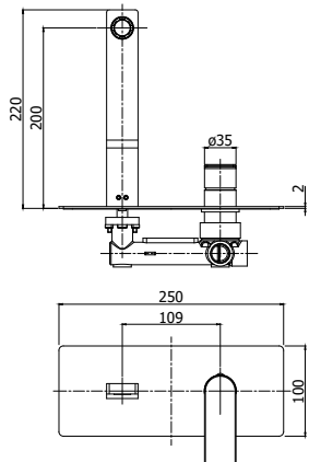
TA 105-104-106CR Miscelatore incasso con bocca erogazione a muro 200 mm / 150 mm / 240 mm Concealed wash basin mixer with wall spout 200 mm / 150 mm / 240 mm
