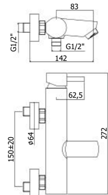
SK 022-023CR Miscelatore vasca doccia con/senza set doccia Bath/shower mixer with/without shower set
