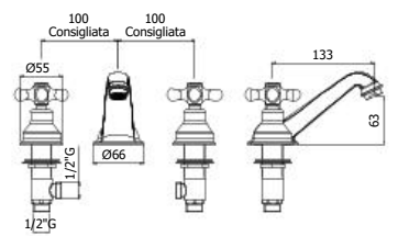
IRV 058CR Batteria lavabo con bocca Retrò Three-hole wash basin mixer with Retrò spout
