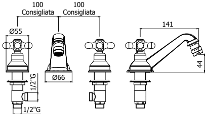
IRV 118CR Batteria bidet con bocca erogazione e scarico Three-hole bidet mixer with spout and pop up waste
