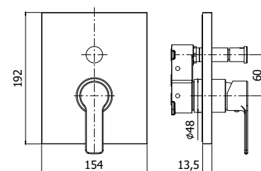
WS BOX015CR Set esterno miscelatore incasso doccia con deviatore External set for concealed shower mixer with diverter
