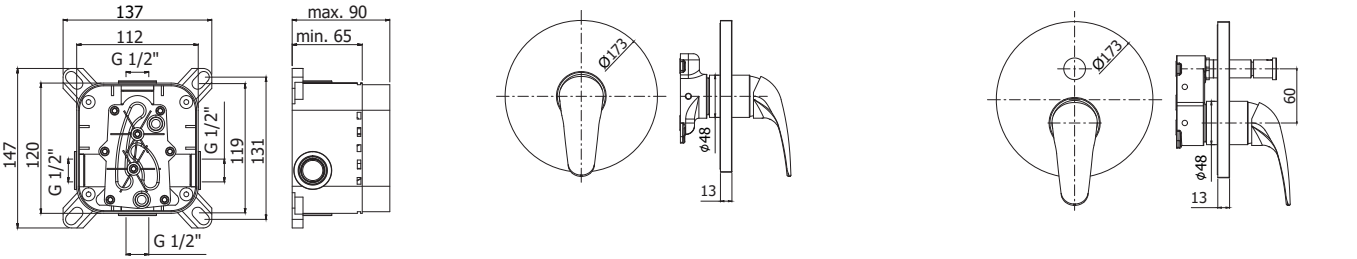
PBOX 001 Set incasso universale per miscelatori doccia Universal Concealed Box for mixers DU BOX010CR Set esterno miscelatore incasso doccia senza deviatore External set for concealed shower mixer without diverter DU BOX015CR Set esterno miscelatore incasso doccia con deviatore External set for concealed shower mixer with diverter
