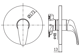
ND BOX010CR Set esterno miscelatore incasso doccia senza deviatore External set for concealed shower mixer without diverter
