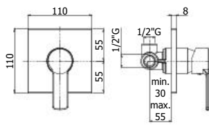
RED 010CR Miscelatore incasso doccia Concealed shower mixer
