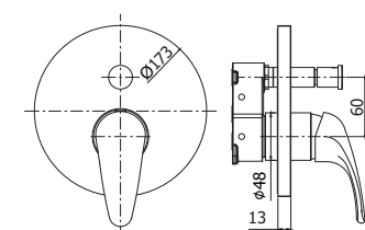
ND BOX015CR Set esterno miscelatore incasso doccia con deviatore External set for concealed shower mixer with diverter
