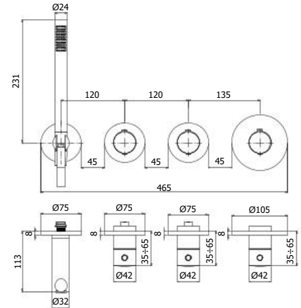
MDE 000 Set esterno per miscelatore termostatico incasso doccia/vasca (2 funzioni) - Installazione solo orizzontale External set for concealed thermostatic shower/bath mixer (2 functions) - Horizontal installation only
