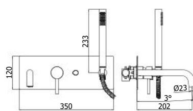
LIG 001CR Miscelatore incasso vasca/doccia completo di deviatore, bocca e set doccia Concealed bath/shower mixer with diverter, spout and shower kit
