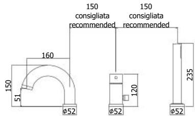
SK 040L-041LCR Miscelatore bordo vasca con doccia estraibile, con/senza bocca erogazione Deck mounted bath mixer with pull out hand-shower, with/without spout
