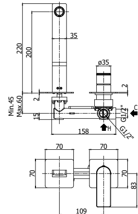
TA 105-104-106CR70 Miscelatore incasso con bocca erogazione a muro 200 mm / 150 mm / 240 mm Concealed wash basin mixer with wall spout 200 mm / 150 mm / 240 mm
