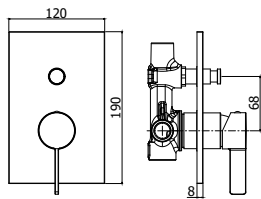
RO 015CR Miscelatore incasso doccia con deviatore Concealed shower mixer with diverter
