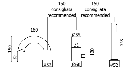
BI 047-048CR MAX FLOW Miscelatore bordo vasca con doccia estraibile, con/senza bocca erogazione Deck mounted bath mixer with pull out hand-shower, with/without spout
