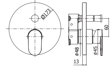
CA BOX015CR Set esterno miscelatore incasso doccia con deviatore External set for concealed shower mixer with diverter
