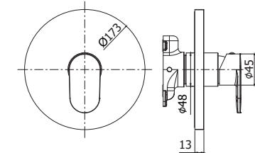
CA BOX010CR Set esterno miscelatore incasso doccia senza deviatore External set for concealed shower mixer without diverter
