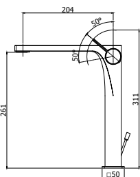
RO 081-085CR Miscelatore lavabo prolungato con senza scarico Tall wash basin mixer with without pop up waste
