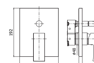
EL BOX015CR Set esterno miscelatore incasso doccia con deviatore External set for concealed shower mixer with diverter
