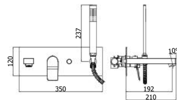
TI 001CR Miscelatore incasso vasca/doccia completo di deviatore, bocca e set doccia Concealed bath/shower mixer with diverter, spout and shower kit
