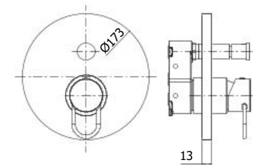
JK BOX015CR Set esterno miscelatore incasso doccia con deviatore External set for concealed shower mixer with diverter
