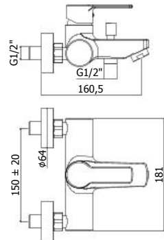
RED 022-023CR Miscelatore vasca/doccia con/senza set doccia Bath/shower mixer with/without shower set
