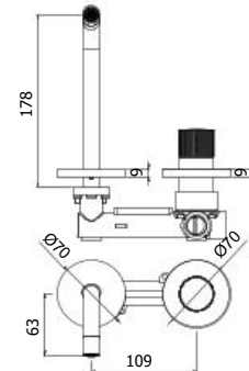
JO 105-104-106CR70 Miscelatore incasso con bocca erogazione a muro 178 mm / 123 mm / 248 mm Concealed wash basin mixer with wall spout 178 mm / 123 mm / 248 mm
