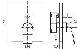
TI BOX015CR Set esterno miscelatore incasso doccia con deviatore External set for concealed shower mixer with diverter
