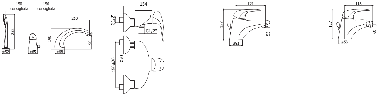
DU 040-041CR Batteria miscelatore bordo vasca con doccia estraibile, con/ senza bocca erogazione Deck mounted bath mixer with pull out hand-shower, with/ without spout DU 168-168DCR Miscelatore doccia con/ senza set doccia Shower mixer with/ without shower set DU 071-075CR Miscelatore lavabo con/ senza scarico Wash basin mixer with/ without pop up waste DU 131-135CR Miscelatore bidet con/ senza scarico Bidet mixer with/ without pop up waste
