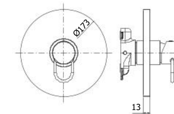
JK BOX010CR Set esterno miscelatore incasso doccia senza deviatore External set for concealed shower mixer without diverter
