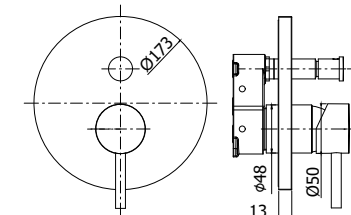
SK BOX015CR Set esterno miscelatore incasso doccia (2 uscite) External set for concealed shower mixer (2 outlets)
