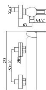
RIN 168-168DCR Miscelatore doccia attacco 1/2\" con senza set doccia Shower mixer 1/2\" connection with without shower set
