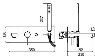
RO 001CR Miscelatore vasca incasso completo di deviatore, bocca e set doccia Concealed bath/shower mixer with diverter, spout and shower kit
