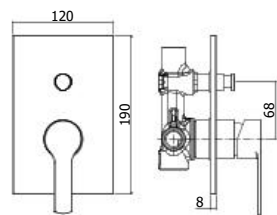
RED 015CR Miscelatore incasso doccia con deviatore Concealed shower mixer with diverter
