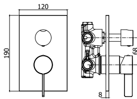
RO 018-019CR Miscelatore incasso doccia con deviatore 2 uscite /3 uscite Concealed shower mixer with diverter 2 outlets /3 outlets
