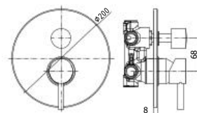
SK 018CR Miscelatore incasso doccia (2 uscite) con cartuccia deviatore Concealed shower mixer (2 outlets) with diverter cartridge
