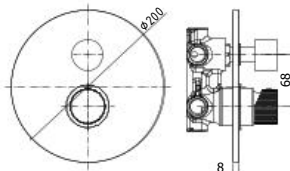
JO 018CR Miscelatore incasso doccia (2 uscite) con cartuccia deviatore Concealed shower mixer (2 outlets) with diverter cartridge
