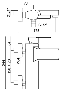
TA 022-023CR Miscelatore vasca doccia con/senza set doccia Bath/shower mixer with/without shower set
