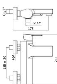
RIN 022-023CR Miscelatore vasca/doccia con senza set doccia Bath/shower mixer with without shower set
