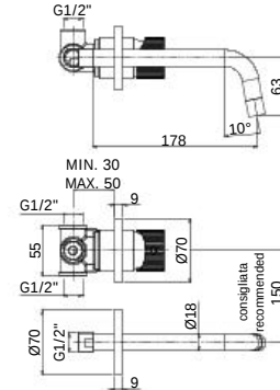
JO 006-007CR70 Miscelatore incasso con bocca erogazione a muro 175 mm / 245 mm Concealed two-hole basin mixer with wall spout 175 mm / 245 mm
