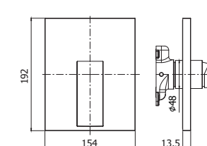
EL BOX010CR Set esterno miscelatore incasso doccia senza deviatore External set for concealed shower mixer without diverter
