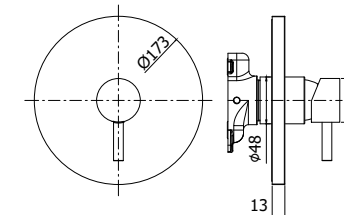
SK BOX010CR Set esterno miscelatore incasso doccia (1 uscita) External set for concealed shower mixer (1 outlet)
