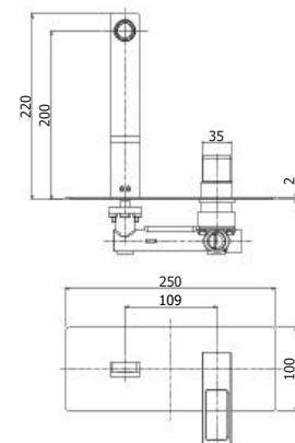
EF 105-104-106CR Miscelatore incasso con bocca erogazione a muro 200 mm / 150 mm / 240 mm Concealed wash basin mixer with wall spout 200 mm / 150 mm / 240 mm
