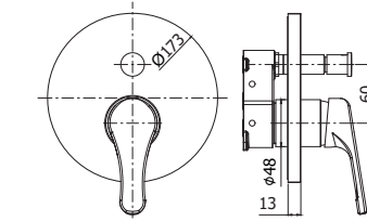
NT BOX015CR Set esterno miscelatore incasso doccia con deviatore External set for concealed shower mixer with diverter
