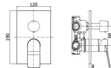
TI 018CR Miscelatore incasso doccia (2 uscite) con cartuccia deviatore Concealed shower mixer (2 outlets) with diverter cartridge
