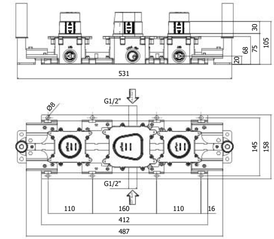
MDBOX 001 Set incasso per miscelatore termostatico doccia/vasca (2 funzioni) - Installazione solo orizzontale Concealed set for thermostatic shower/bath mixer (2 functions) - Horizontal installation only
