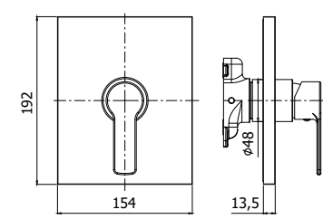
WS BOX010CR Set esterno miscelatore incasso doccia senza deviatore External set for concealed shower mixer without diverter
