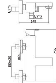
EF 022-023CR Miscelatore vasca doccia con/ senza set doccia Bath/shower mixer with/ without shower set
