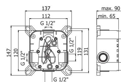
PBOX 001 Set incasso universale per miscelatori doccia Universal Concealed Box for mixers bath
