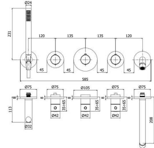
MDE 001 Set esterno per miscelatore termostatico incasso doccia/vasca (2 funzioni) - Installazione solo orizzontale External set for concealed thermostatic shower/bath mixer (2 functions) - Horizontal installation only
