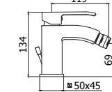
LES 131-135CR Miscelatore bidet con/senza scarico Bidet mixer with/without pop up waste
