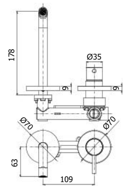
SK 105-104-106CR70 Miscelatore incasso con bocca erogazione a muro 178 mm / 123 mm / 248 mm Concealed wash basin mixer with wall spout 178 mm / 123 mm / 248 mm
