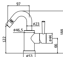
BI 138-137CR Miscelatore bidet con canna orientabile con/ senza scarico Bidet mixer with swivelling spout with/ without pop up waste
