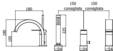
TA 040-041CR Batteria miscelatore bordo vasca con doccia estraibile, con/senza bocca estribile Deck mounted bath mixer with pull out hand-shower, with/without spout
