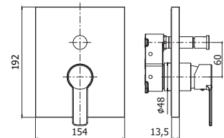
RED BOX015CR Set esterno miscelatore incasso doccia con deviatore External set for concealed shower mixer with diverter
