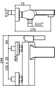
RO 022-023CR Miscelatore vasca doccia con senza set doccia Bath/shower mixer with without shower set
