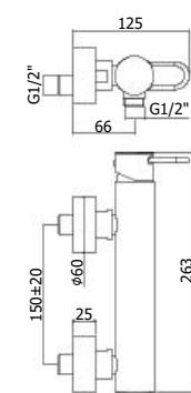
JK 168-168DCR Miscelatore doccia esterno attacco 1/2" con/ senza set doccia Shower mixer 1/2" connection with/ without shower set
