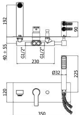
RED 001CR Miscelatore vasca incasso completo di deviatore, bocca e set doccia Concealed bath/shower mixer complete with diverter, spout and shower kit
