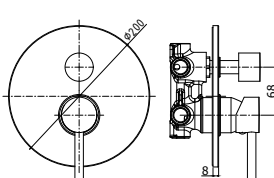
BI 019CR Miscelatore incasso doccia (3 uscite) con cartuccia deviatore Concealed shower mixer (3 outlets) with diverter cartridge
