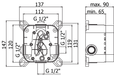
PBOX 001 Set incasso universale per miscelatori doccia Universal Concealed Box for mixers doccia
