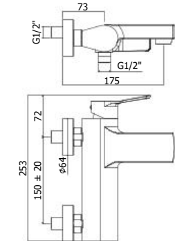
TI 022-023CR Miscelatore vasca doccia con/senza set doccia Bath/shower mixer with/without shower set
