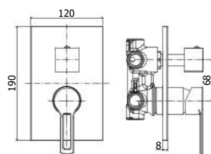
RIN 018-019CR Miscelatore incasso doccia con deviatore 2 uscite /3 uscite Concealed shower mixer with diverter 2 outlets /3 outlets
