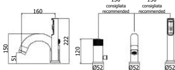
JO 040L-041LCR Miscelatore bordo vasca con doccia estraibile, con/senza bocca erogazione Deck mounted bath mixer with pull out hand-shower, with/without spout
