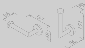
Toiletrolhouder / Reserverolhouder Toilet roll holder / Spare toilet roll holder 916509-10
