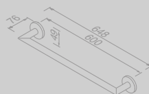
Handdoekrek 60 cm Towel rail 60 cm
