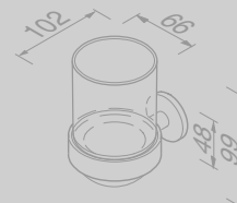
Glashouder met glas Glass holder with glass 916502-10
