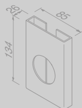
Houder voor hygiënische zakjes Hygienic bag dispenser
