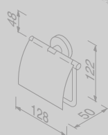
Toiletrolhouder met klep Toilet roll holder with cover 916508-10
