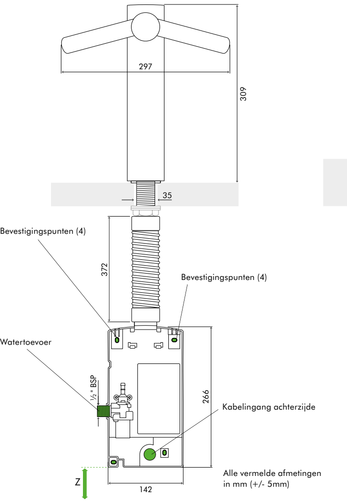
ACHTERAANZICHT
