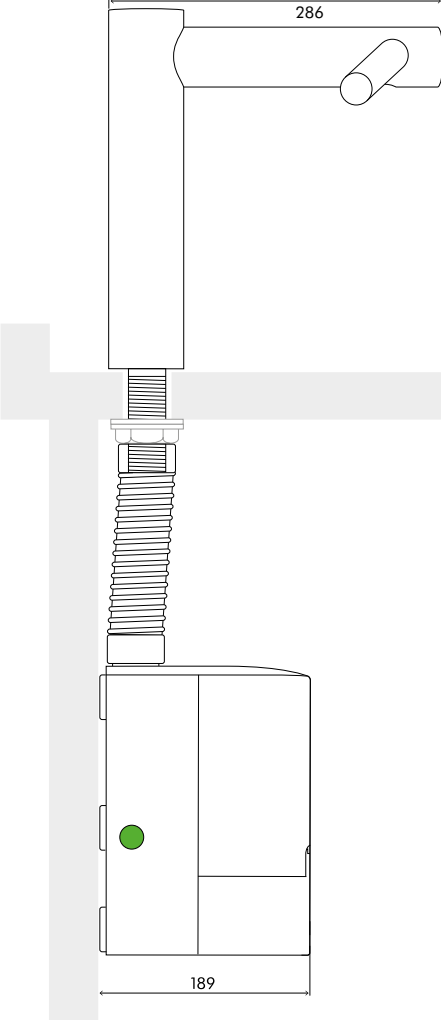
ZIJAANZICHT
